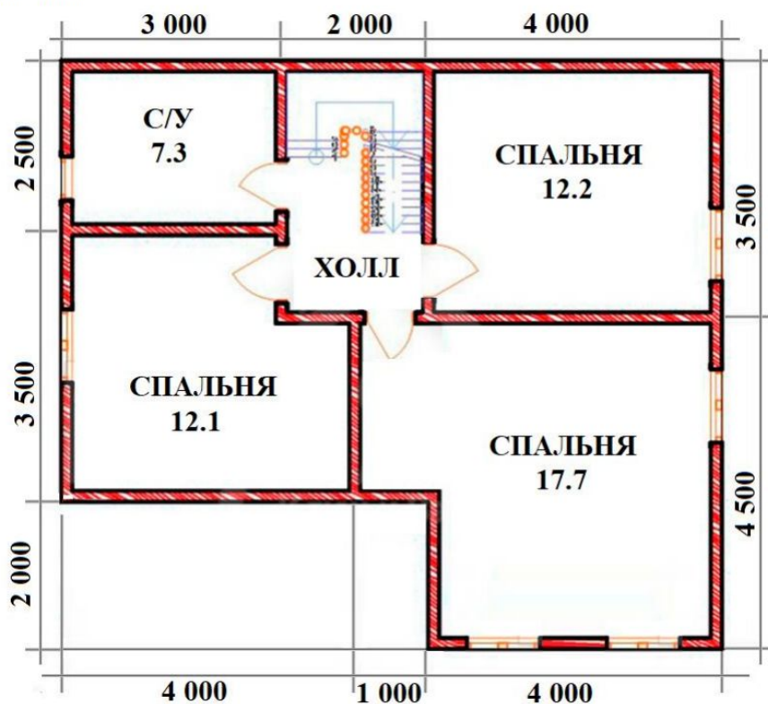
План 2 этажа:
