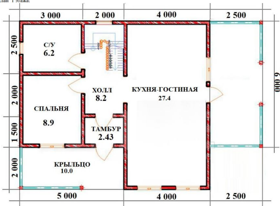
План 1 этажа:
