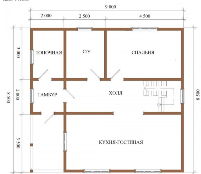
План 1 этажа:
