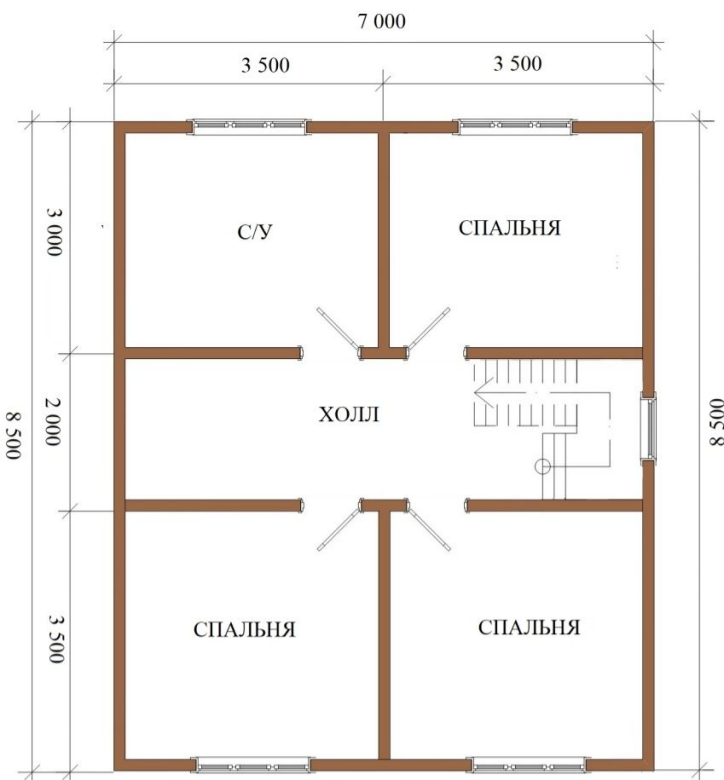
План 2 этажа:
